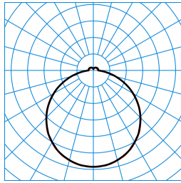
Olisq Act QWD3 DW 30 ETDD8 IP54 IK (ActDSU) TX375897
