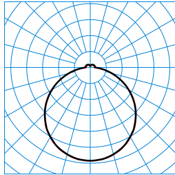
Olisq Act QWD3 DW 30 ETDD8 IP54 IK (ActDCW) TX375867
