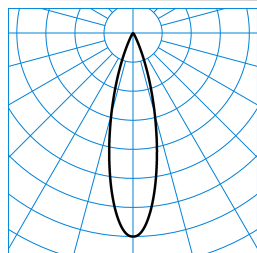
E-Line 7651 LentyP L-MF 20-EC M39 ET 05 (150) TX463317
