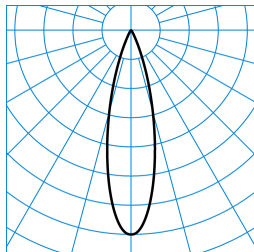
E-Line 7651 LentyP L-MF 20-827 M32 ET 03 (225) TX463368
