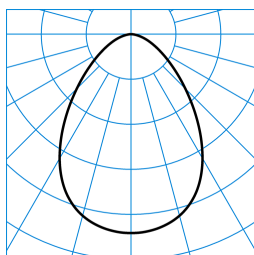
InperiaLP C05 BR22 1000-840 01 + DA-M 01 TX371223 ■ C0 - C180
