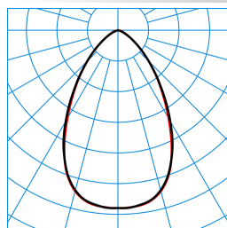
Mirona Fit TB LED17000-865 TX280653
