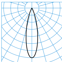
E-Line 7651 Lentyp L-MF 30-BF M54 ET 01 (225) TX463276
