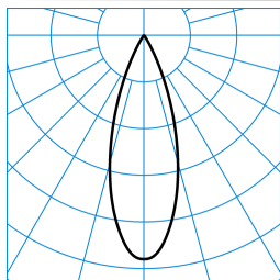
E-Line 7651 LentyP L-FL 40-EW M48 ETDD 05 (150) TX463157
