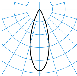
E-Line 7651 LentyP L-FL 40-EW M48 ETDD 05 (225) TX463158
