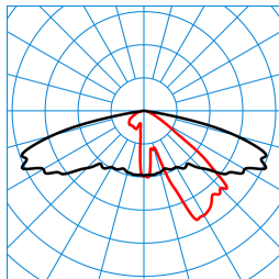
Publisca P1W-AB2L-LR/1800-740 2G1S ET (CLO initial value) TX300289
