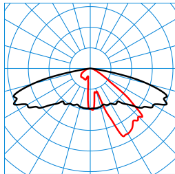
Publisca P1W-AB2L-LR/1800-740 2G1S ET (CLO end value) TX301705
