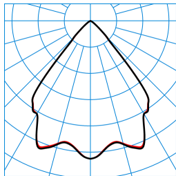
Creavo M48-TS LW19-03 62-830 ET 01 TX372015
