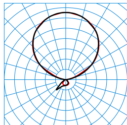
LuceoS S-U PAW-IL 300-840 05(LEO2) TX371970
