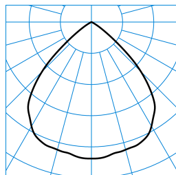
InperiaL G2 C07 HR22 2700-840 03 + DA 03 TX053092 ■ C0 - C180
