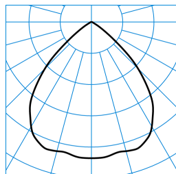
InperiaL G2 C07 HR22 2700-840 03 + RD-PC TX053094 ■ C0 - C180
