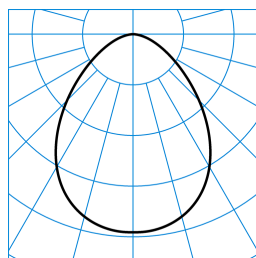
InperiaL G2 C07 HR22 2700-840 03 + DA-M 03 TX053093 ■ C0 - C180
