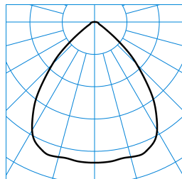
InperiaL G2 C07 HR22 2700-840 03 + ZN-PC TX053096 ■ C0 - C180
