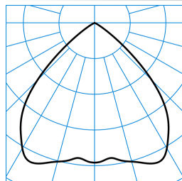
InperiaL G2 C07 HR22 2700-840 03 TX053091 ■ C0 - C180
