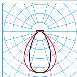
Tugra 18 PN 70-840 ET PC 23 TX302913
