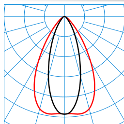
Mirona Fit T LED26000-840 ESG TX050473
