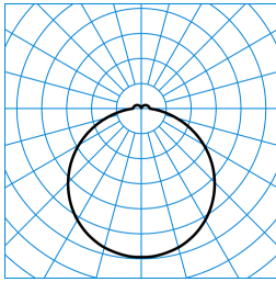
Olisq RWD3 DW 50-830 ETBLE +DMR PC + Olisq RWD3 ZDR 1/2 03 TX429100
