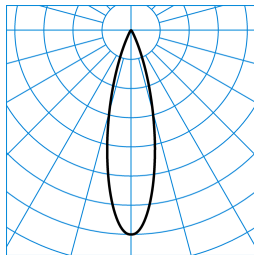
E-Line 7651 LentyP L-MF 40-827 M32 ETDD 05 (225) TX463386
