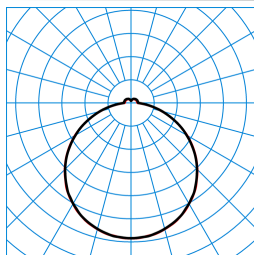
Olisq QWD3 DW 45-830 ET IP54 IK TX375707
