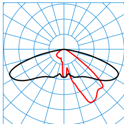
Publisca P1-AB2L-LR/4600-740 6G1S ET (CLO initial value) TX300953 ■ C0 - C180 ■ C90 - C270 DIN 5040: A30 UTE: 1,00 G CEN Flux Code: 35 74 97 100 100
