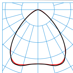
Mirona Fit B LED17000-865 TX280682
