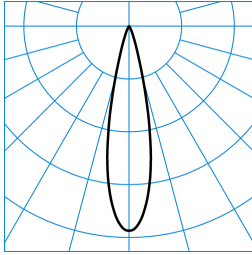
E-Line 7651 LentyP L-SP 30-835 M34 ET 01 (225) TX463648
