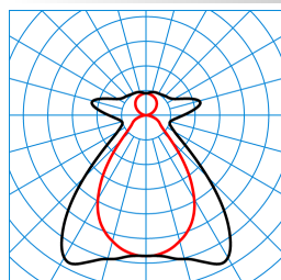
TugraHE 12 PW19-IL 45-840 ETDD C2 TX306464
