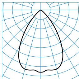
InperiaL G2 C07 HR22 3800-840 ET 03 ■ C0 - C180 TX373471
