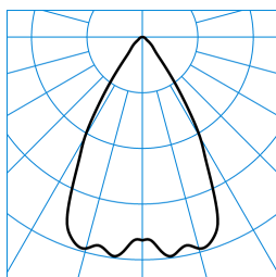
InperiaLP C05 HR19 1000-840 03 + RG-PC ■ C0 - C180 TX369787
