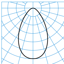
InperiaLP C05 HR19 1000-840 03 + DA-M 03 ■ C0 - C180 TX369785
