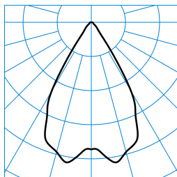
InperiaLP C05 HR19 1000-840 03 + ZN-PC ■ C0 - C180 TX369788
