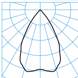
InperiaLP C05 HR19 1000-840 03 ■ C0 - C180 TX369781
