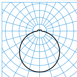
Olisq RWD3 DW 30-840 ET IP54 PC TX375877
