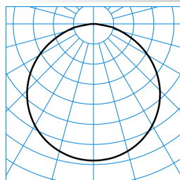
Skeo Circ MultiLC WD2 1G1Y ETDD (ww) ■ C0 - C180 TX059430
