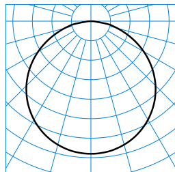
Skeo Circ MultiLC WD2 1G1Y ETDD (cw) ■ C0 - C180 TX278652
