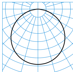
Skeo Circ MultiLC WD2 1G1Y ETDD (nw) ■ C0 - C180 TX278655
