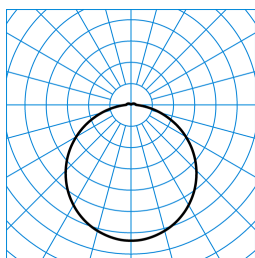
Olisq RWD3 DW 50-830 ET HFS IP54 PC + Olisq RWD3 C 01 TX426479
