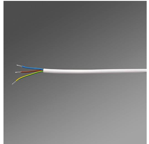
A-LTG 2300 3x0,75
