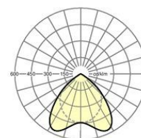
Lichttechniek Micro-paraboolrooster gesatineerd-direct stralend HLHX/1500 LED 4000 lm 840
