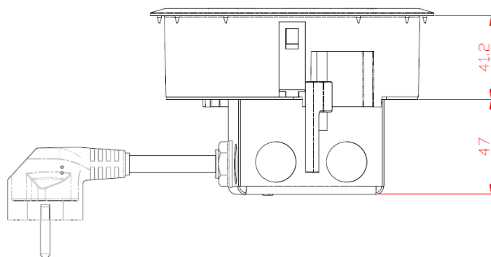
Zijaanzicht vloerdoos
