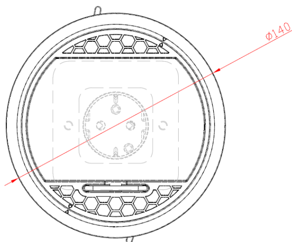
Bovenaanzicht vloerdoos
