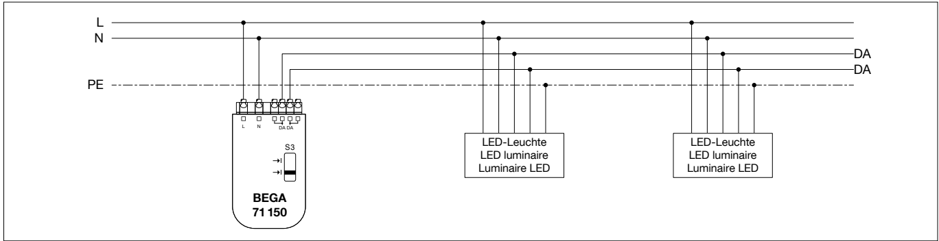
Schaltbild Betriebsart 2
