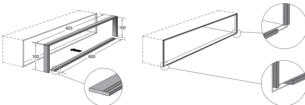
Einbau in waagrechter Brennlage · Installation in horizontal mounting position · Installation en position horizontale
