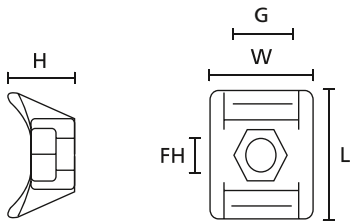
NY3256 (zijaanzicht)
