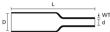
Krimpkous 3:1
