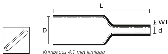
Krimpous 4:1 met lijmlaag
