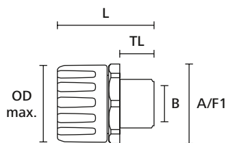
HelaGuard koppeling, recht met niet-draaiend buitendraad
