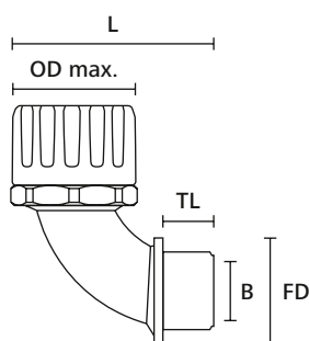
HelaGuard koppeling, 90° met niet-draaiend buitendraad
