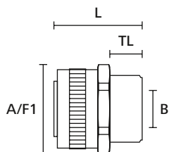
HelaGuard koppeling, recht met niet-draaiend buitendraad
