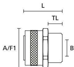
HelasGuard koppeling, recht met niet-draaiend buitendraad
