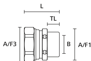
HelaGuard compressiekoppeling, recht met niet-draaiend buitendraad
