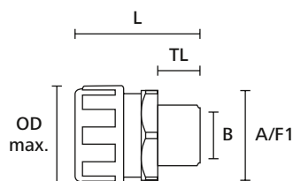
HelaGuard koppeling, recht met niet-draaiend buitendraad
