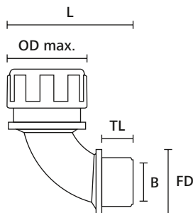
HelaGuard koppeling, 90° met niet-draaiend buitendraad
