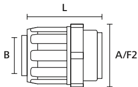
FlexiGuard koppeling, recht met draaiend buitendraad
