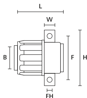
FlexiGuard koppeling, recht met flens
