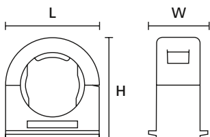
HelaGuard slangklem (zij aanzichten)
