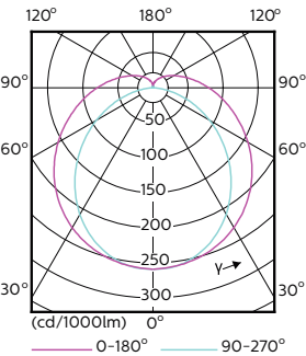
LEDtube 1200mm 26W G5
