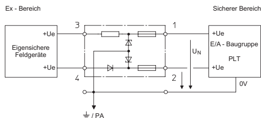
Zwei-Kanal-Sicherheitsbarrieren Sicherheitsbarriere Potential: + / Auswertebaugruppe Potential: +
