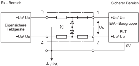
Zwei-Kanal-Sicherheitsbarrieren Sternbarriere / Sternbarriere
