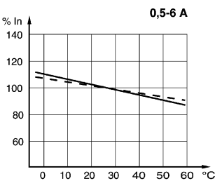
Korrekturfaktoren für die von 30 °C abweichenden Umgebungstemperaturen
