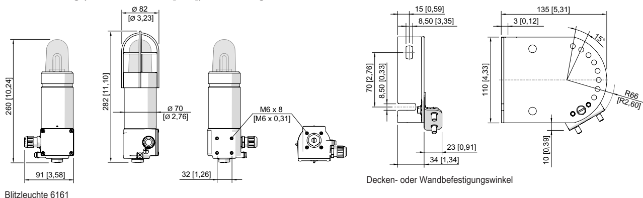
Blitzleuchte 6161
