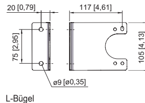
L-Bügel
