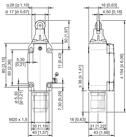
Rollenstößel 8074/2-5-R-40
